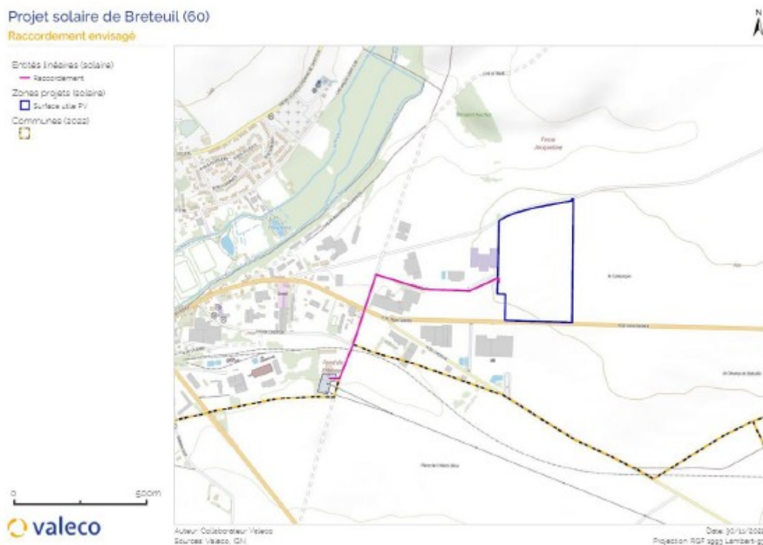
Raccordement prévisionnel au poste source (étude d'impact, figure 6 page 17)
